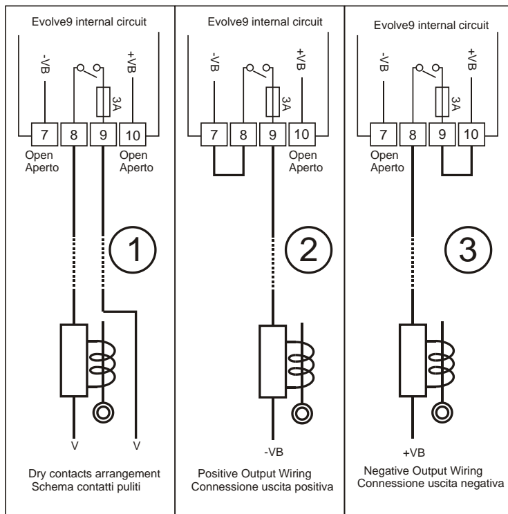
Figura 2: possibilità di connessione della uscita elettrostop (vedi sezione 9.3 per la programmazione)
